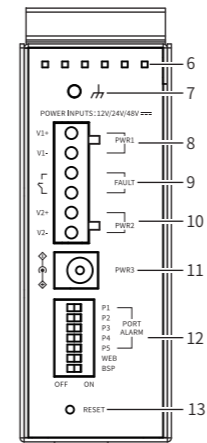
TL-SG1005工业级 上面板示意图
