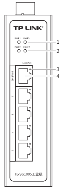
TL-SG1005工业级 前面板示意图
