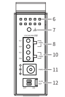
TL-SF1005工业级 上面板示意图
